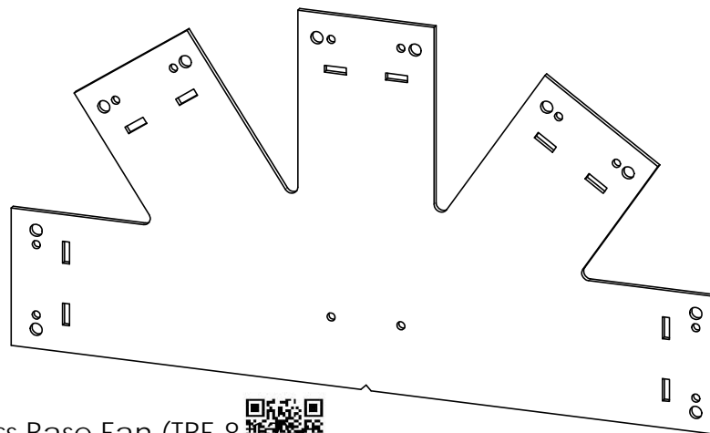
8:12 Truss Base Fan (TBF-8) 56619
